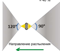
Пример характеристик асимметричной двойной плоскоструйной форсунки с системой впуска воздуха (Lechler IDTA)
