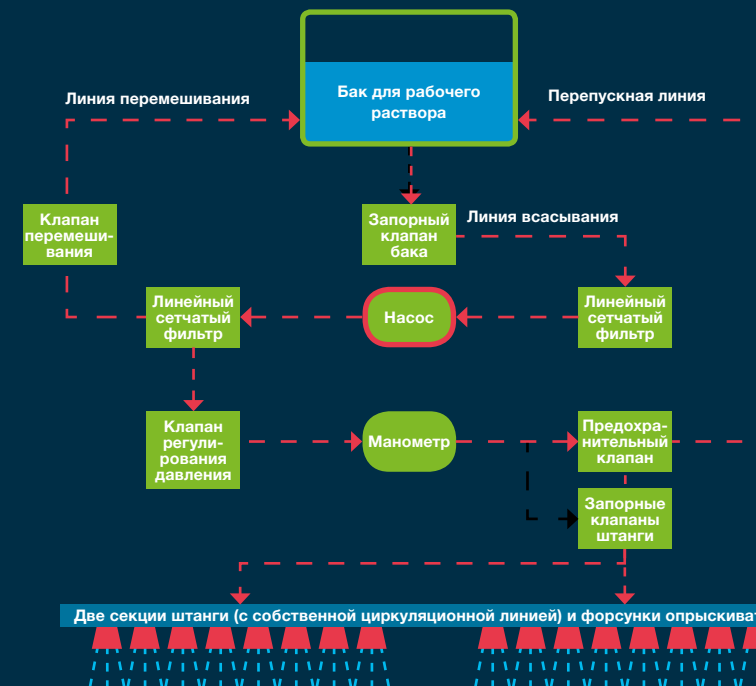
Базовая блок-схема типичного штангового опрыскивателя низкого давления
