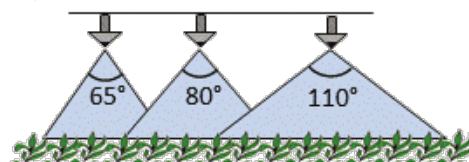
Углы распыления плоскоструйной форсунки
